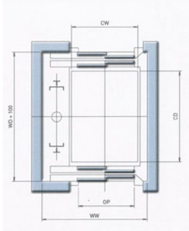
Disposizione in vano in muratura con doppia apertura
