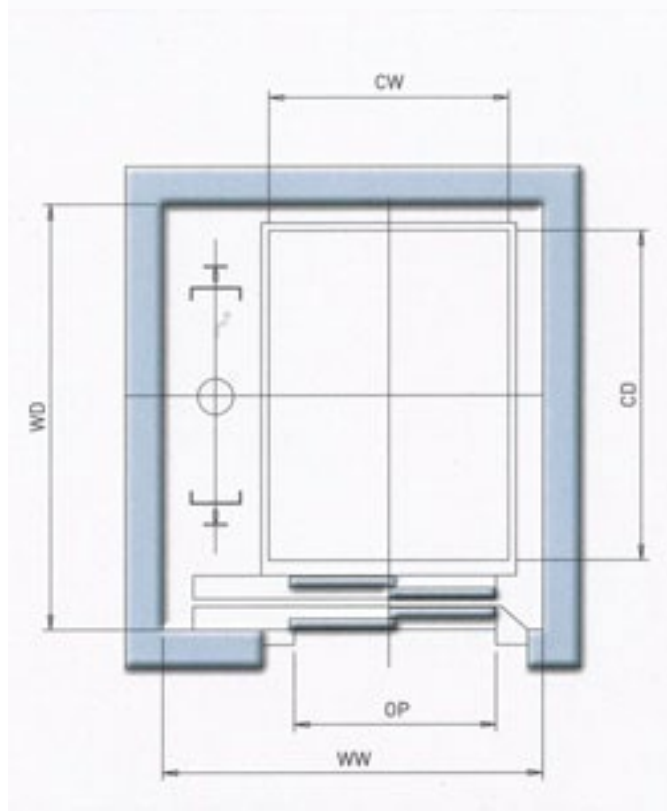
Disposizione in vano in muratura con una apertura
